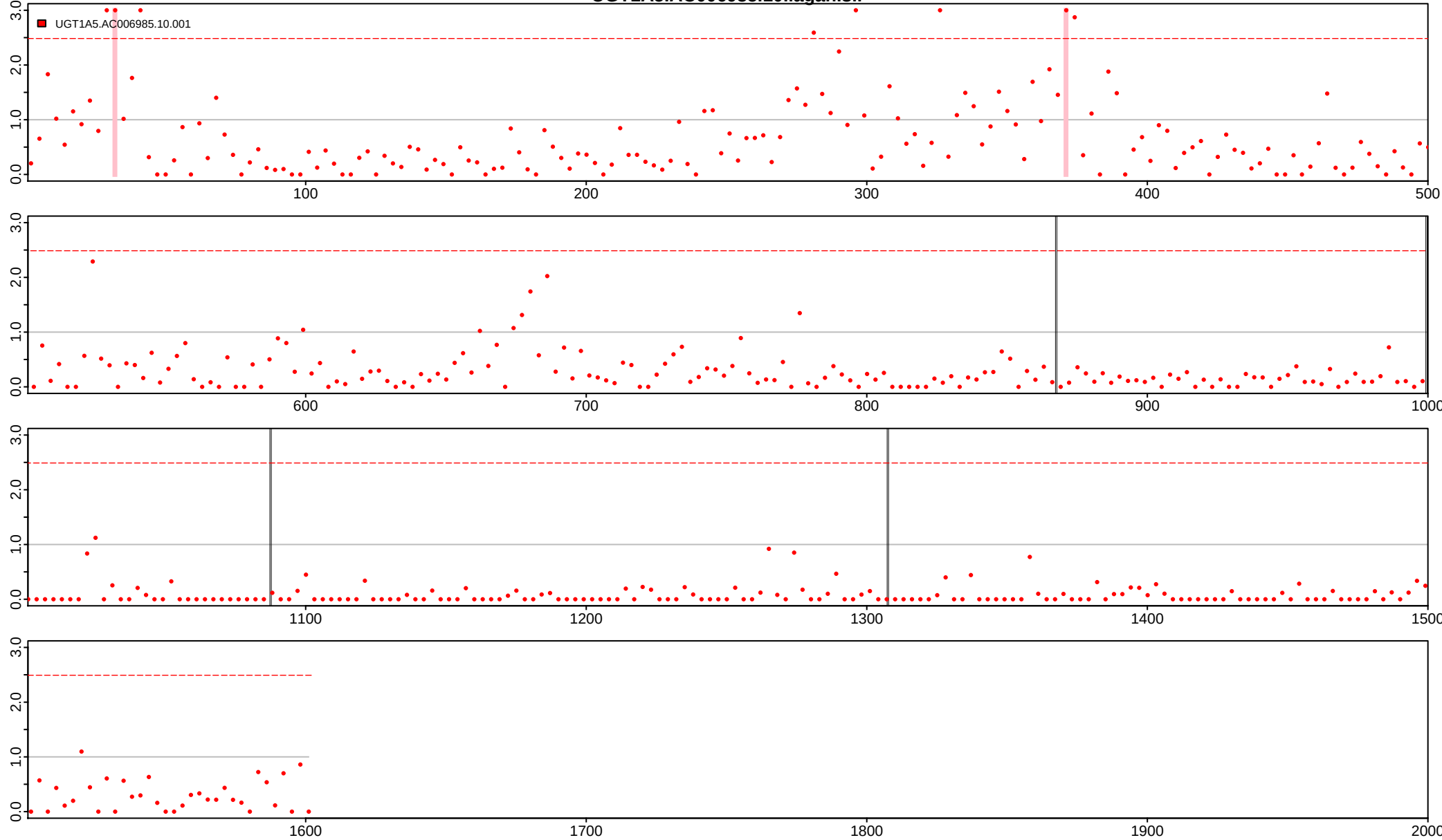
UGT1A5.AC006985.10.lagan.slr
