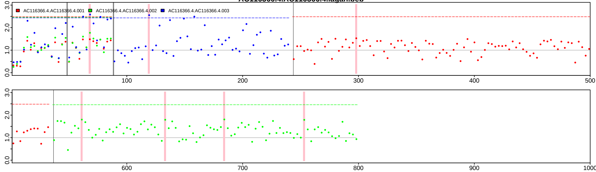
AC116366.4.AC116366.4.lagan.beb
